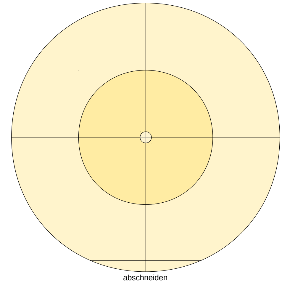
Blende vor dem Filterhalter Flugzeugsperrholz 2 mm
