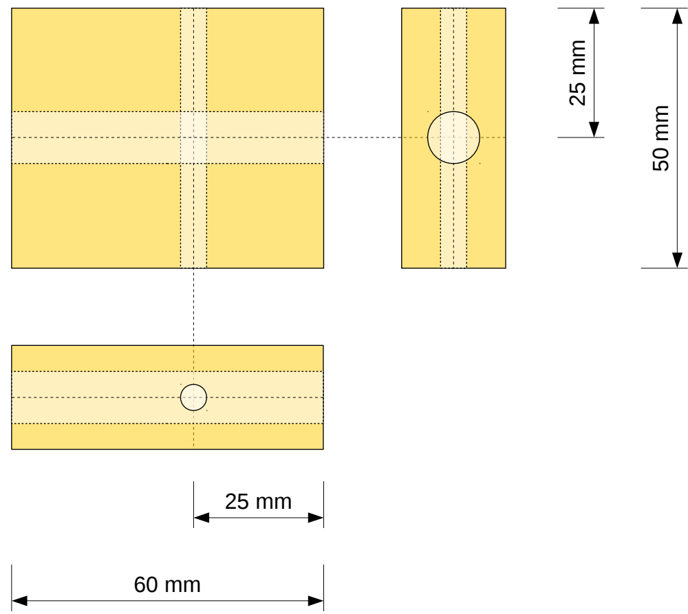
Bohrhilfe für Hutstangen Birke oder Buche Multiplex 20..30 mm
