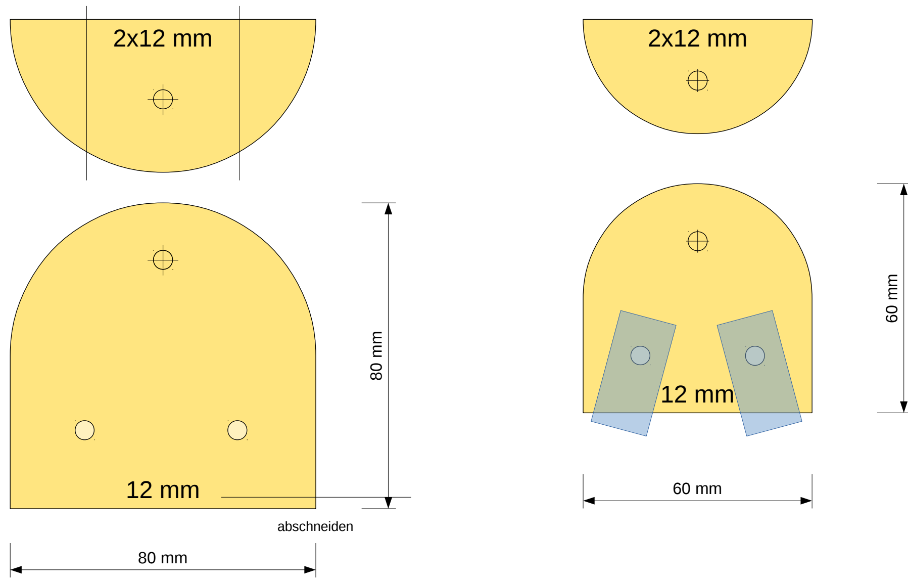
Klemmung am Hut für Stangen Birke Multiplex 12 mm
