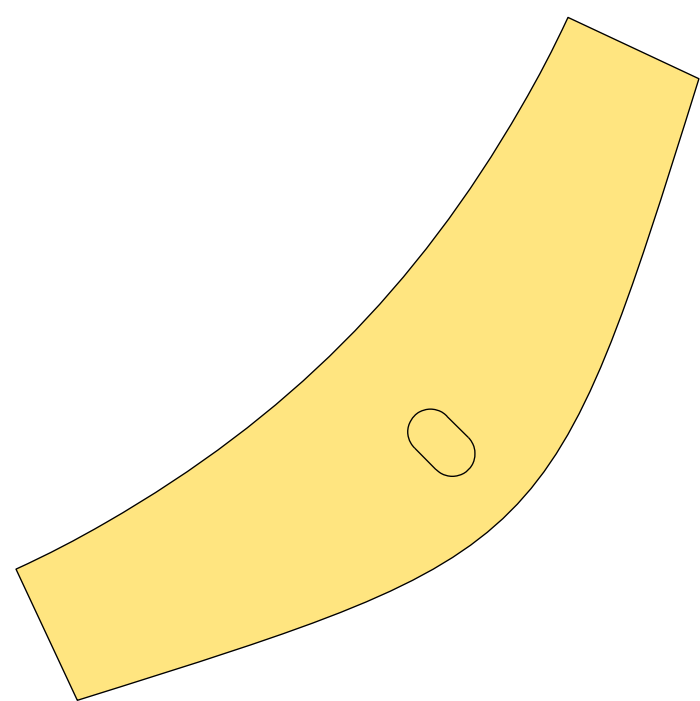
Spiegel Lateralhalterung Birke Multiplex 2x12 mm
