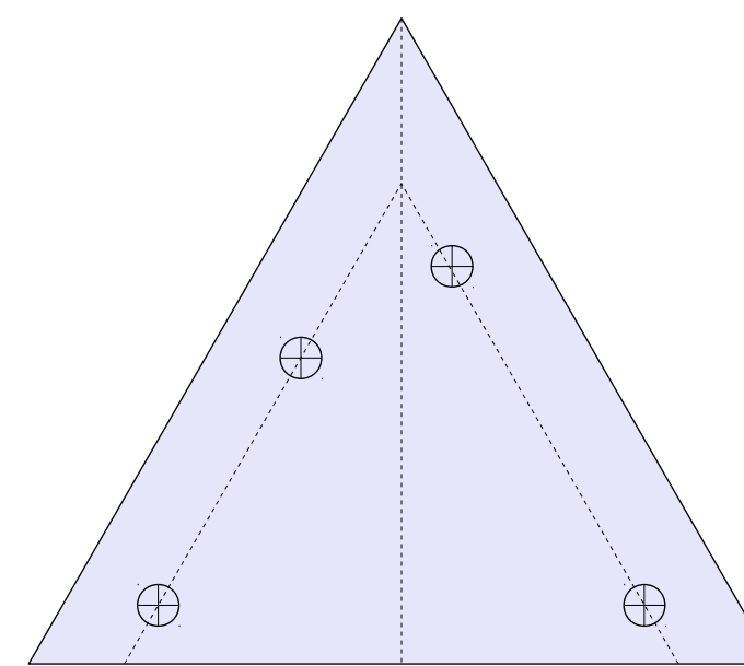
Stützdreieck für die Streben der Spiegelzelle Aluminium 1,5 mm, 3x
