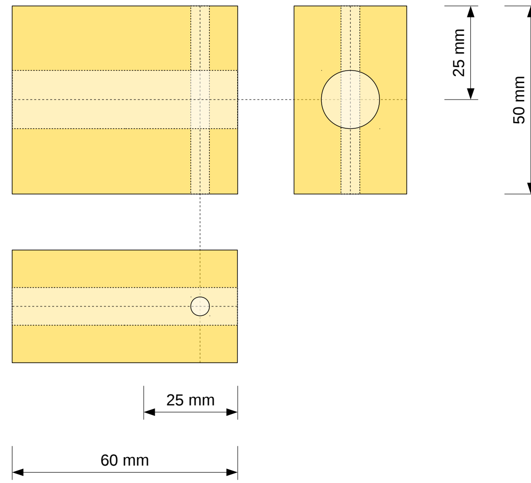
Bohrhilfe für Stangen Birke oder Buche Multiplex 20..30 mm
