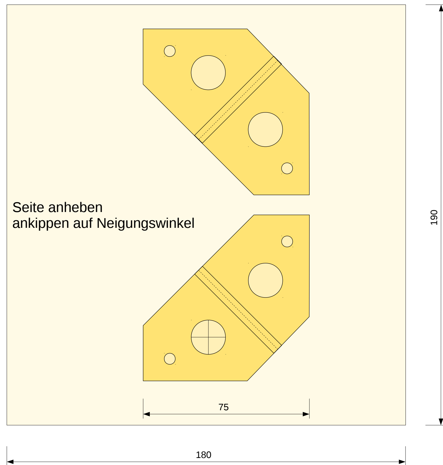
Bohr- und Fräshilfe für untere Blöcke
